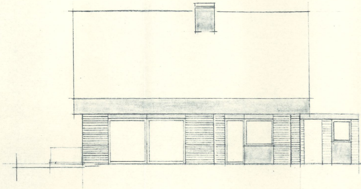
GARTENANSICHT
