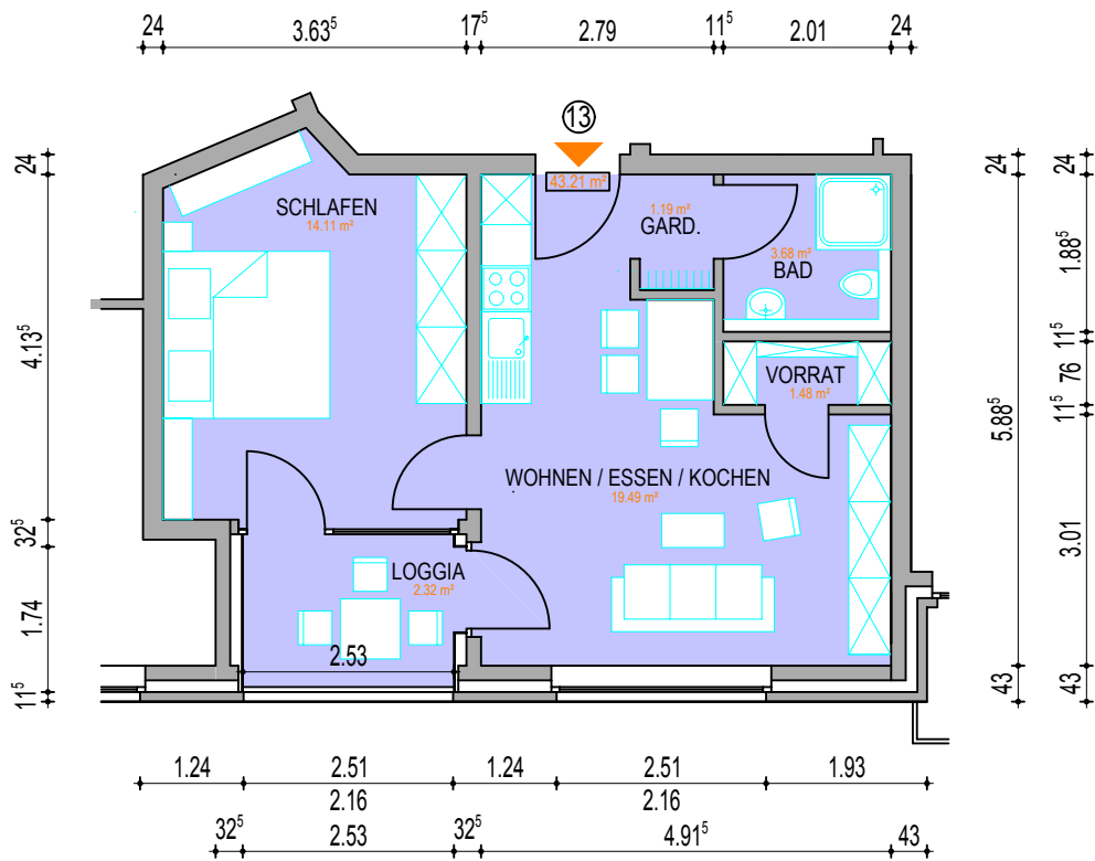
WOHNUNG NR. 13 3. OBERGESCHOSS M. 1:100
