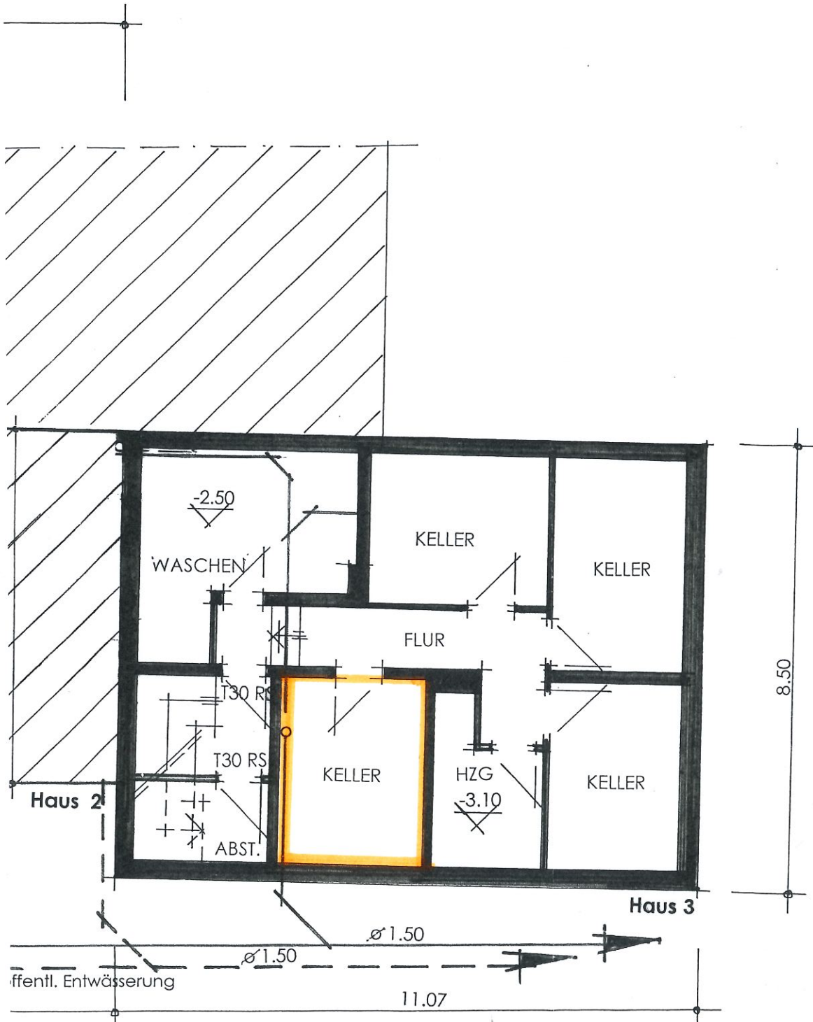
KELLERGESCHOSS IM MASSTAB 1:100
