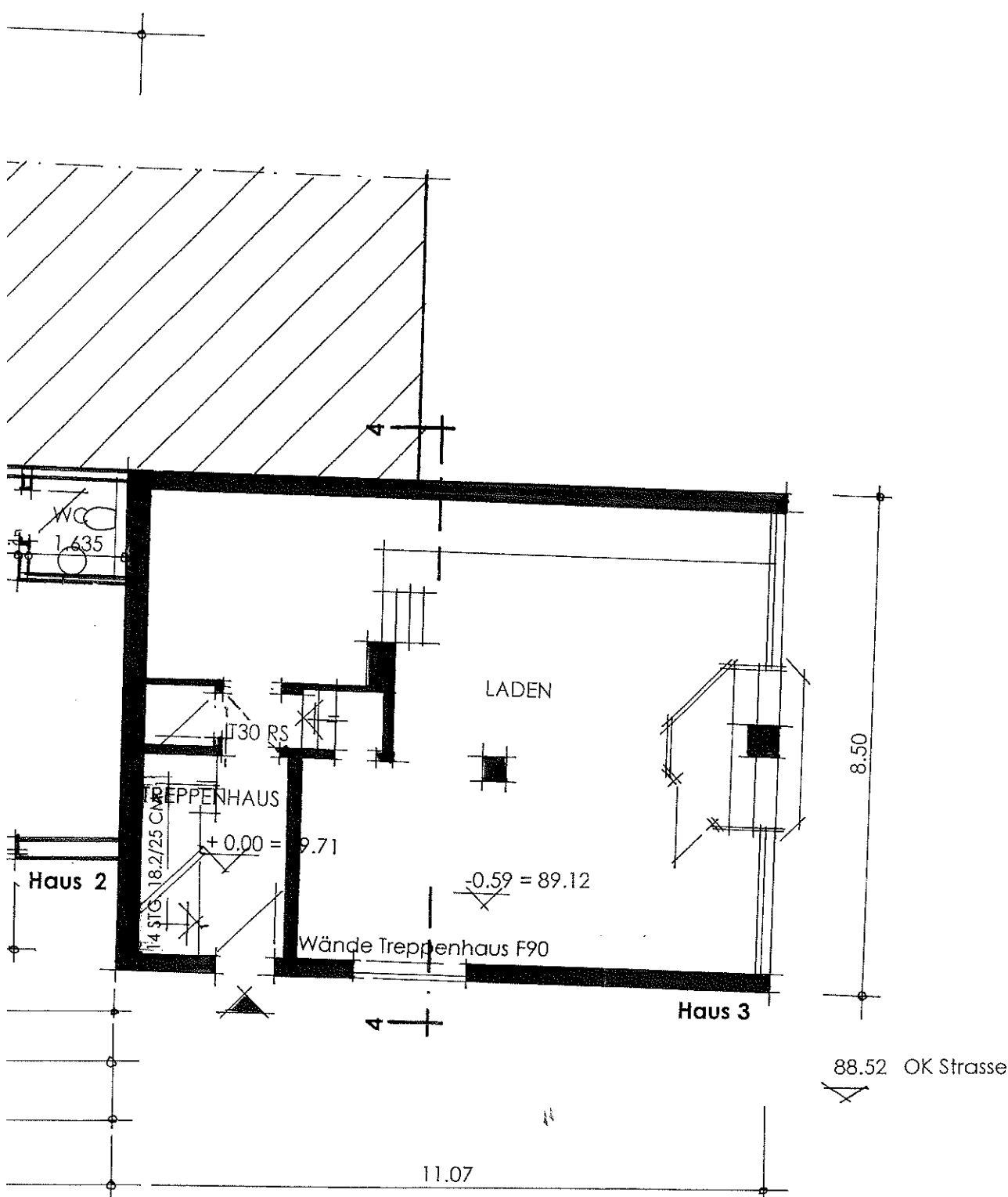
ERDGESCHOSS IM MASSTAB 1:100
