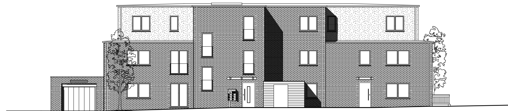
ANSICHT HAUS 1 - OSTEN
