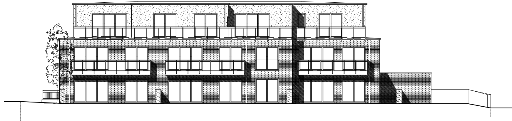
ANSICHT HAUS 1 - WESTEN
